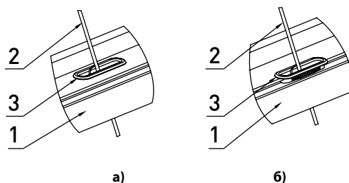
Рис. 44. Установка вставки:
