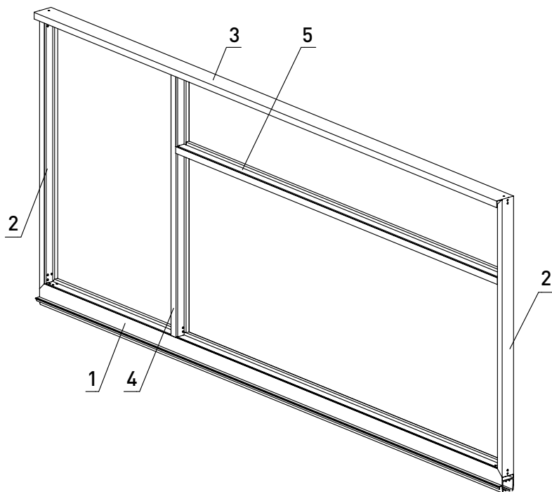
Рис. 2. Рама ворот:
